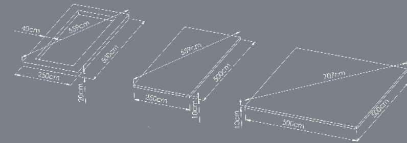
PLAN DE RÉSERVATION MAÇONNERIE
