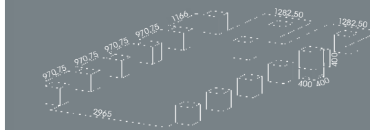
RÉSERVATIONS PLOTS BETON (Cotes en mm)
