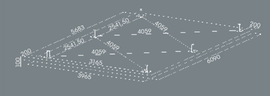
RÉSERVATIONS PLOTS BETON (Cotes en mm)
