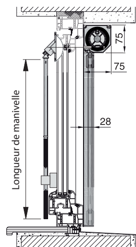
Coffre à pan coupé avec treuil à manivelle (renvoi intérieur 90°)
