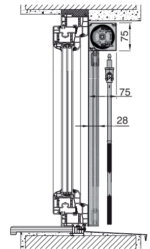
Coffre carré avec treuil à manivelle magnétique amovible (sous caisson)
