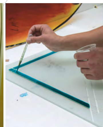
Résicolor® : mise en couleur
