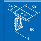
Supporto Bracket
