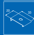
Attacco a scomparsa Hidden bracket
