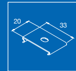
Attacco a scomparsa Hidden bracket
